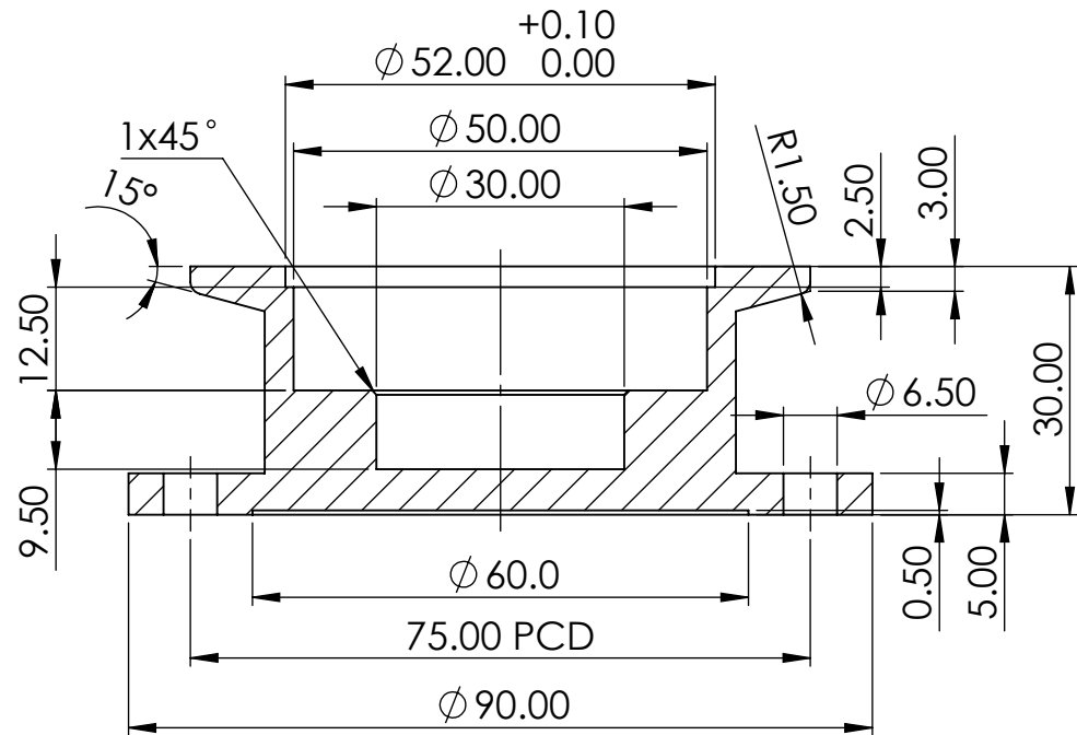
SECTION D-D
